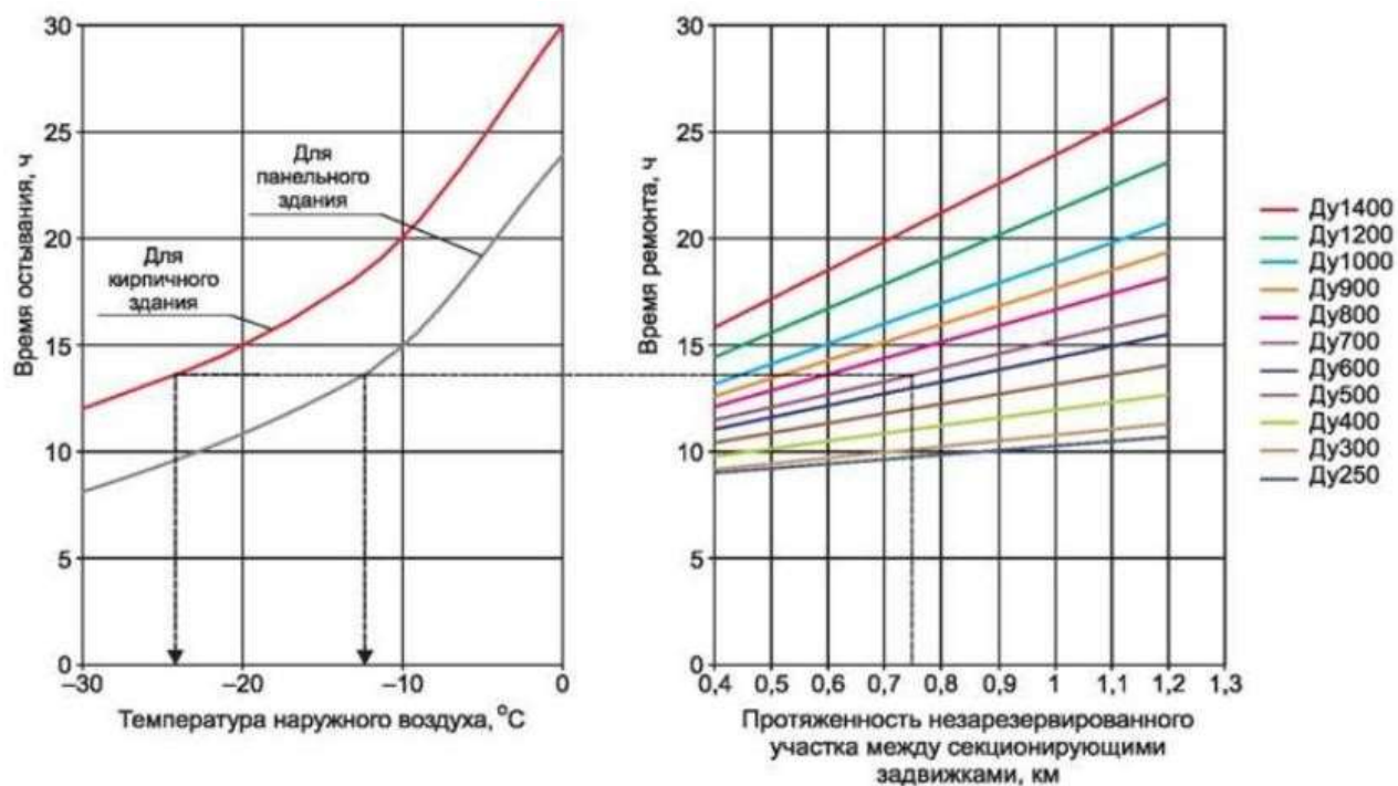
Рисунок 1.5.2 - Номограмма для определения периодов остывания для подъездов и лестничных клеток жилых зданий со снижением температуры с +15 до +3 °C
