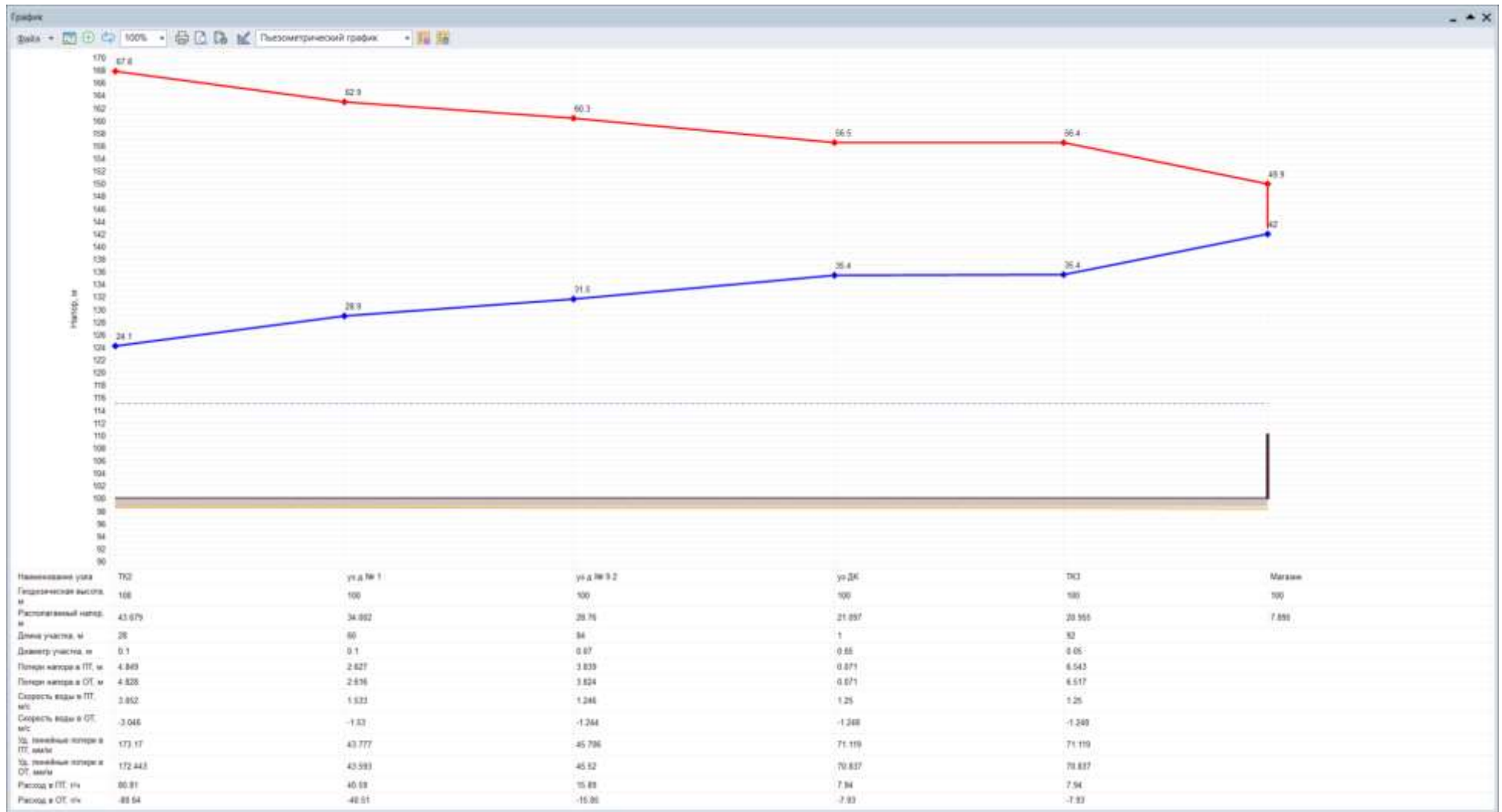
Рисунок 1.3.8 – Пьезометрический график с учетом резервного трубопровода
