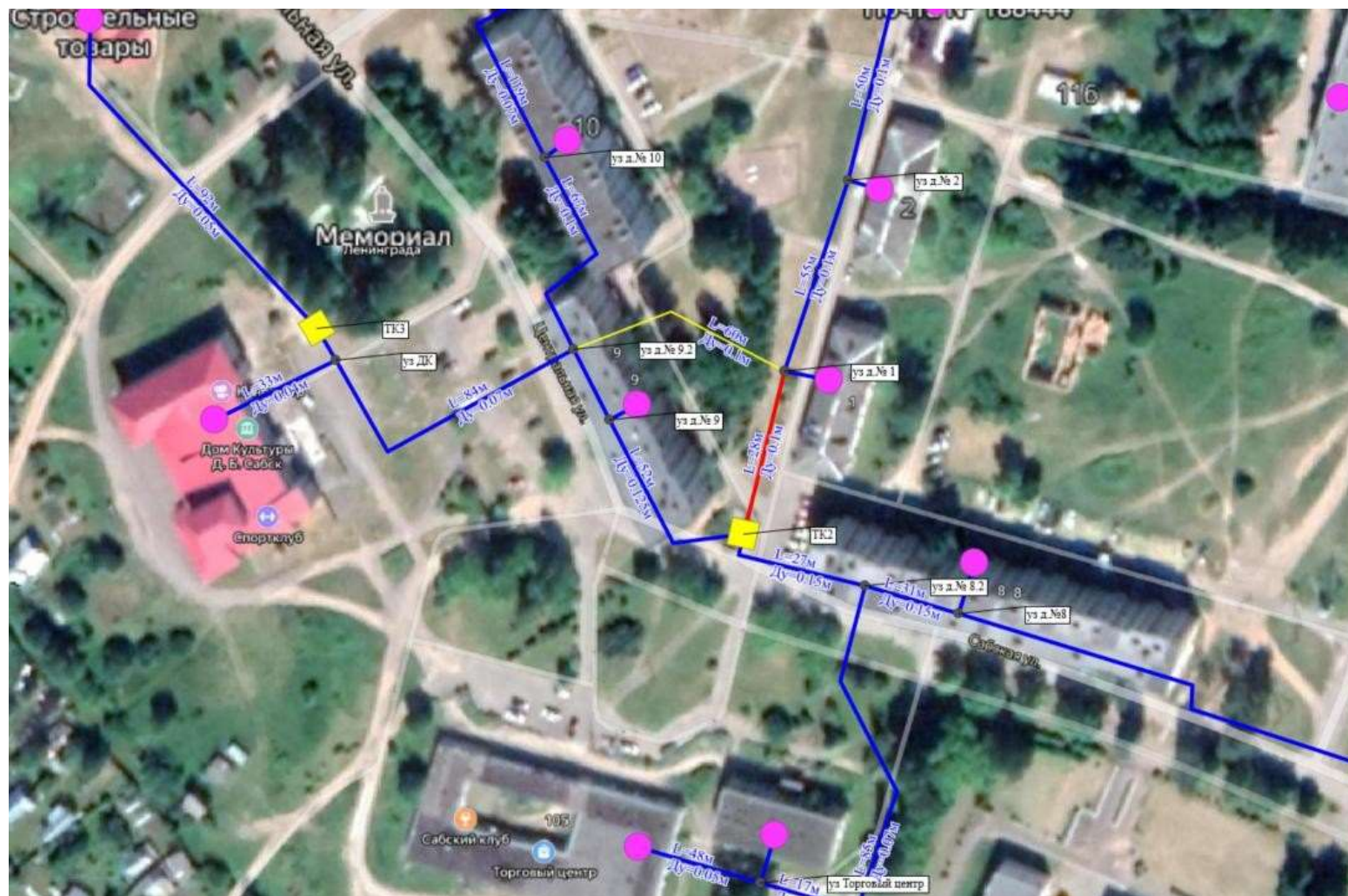
Рисунок 1.3.2 – Резервная перемычка Ду100 мм Уз д.№9.2 - Уз д.№1 – 60 м.
