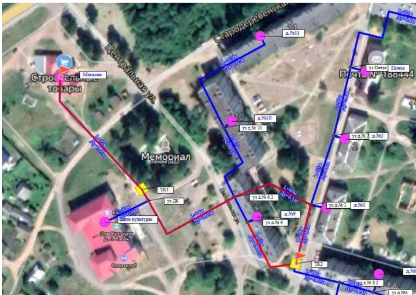
Рисунок 1.3.7 – Путь для построения пьезометрического графика с учетом резервного трубопровода
