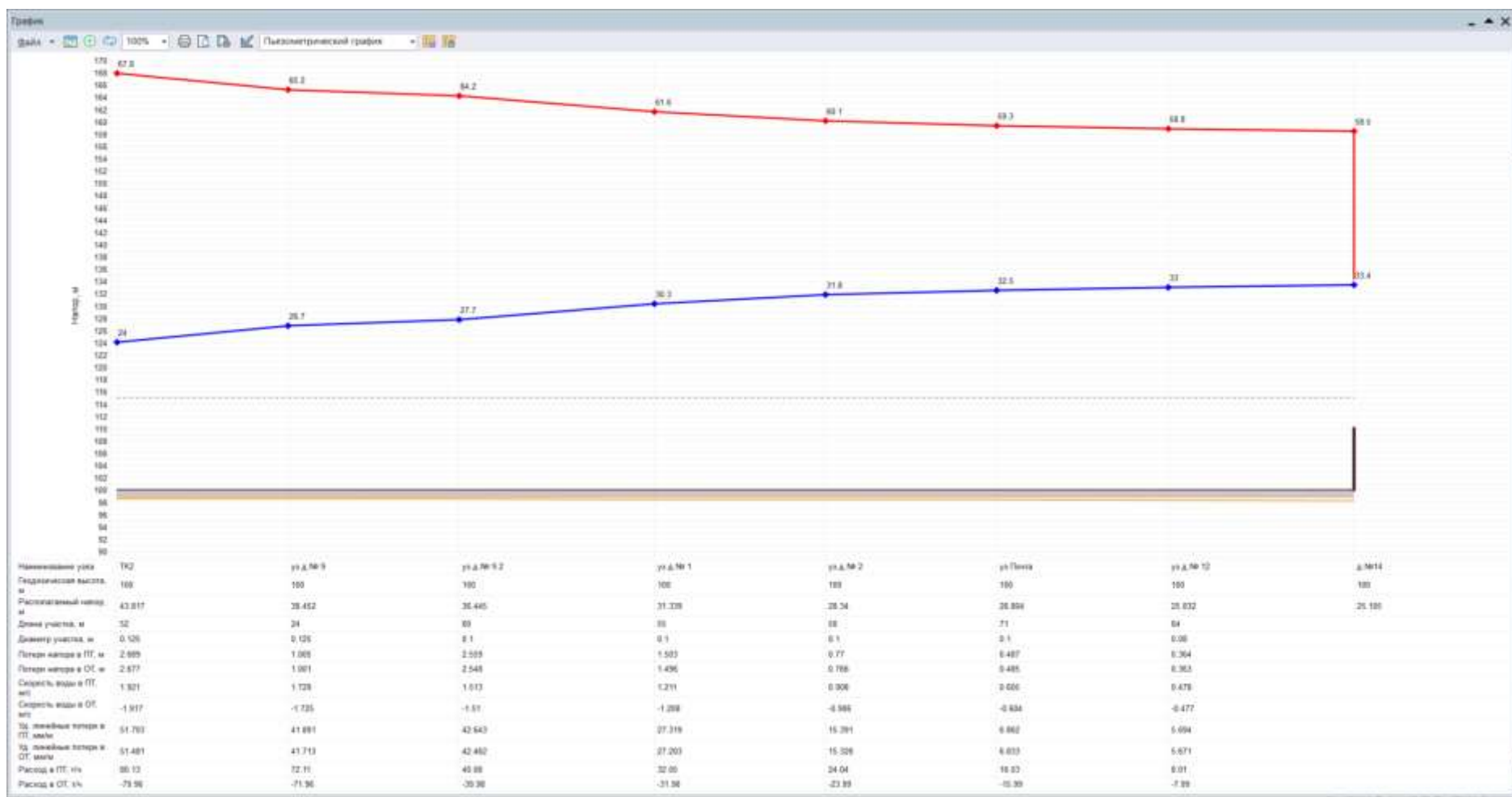
Рисунок 1.3.4 – Пьезометрический график с учетом резервного трубопровода
