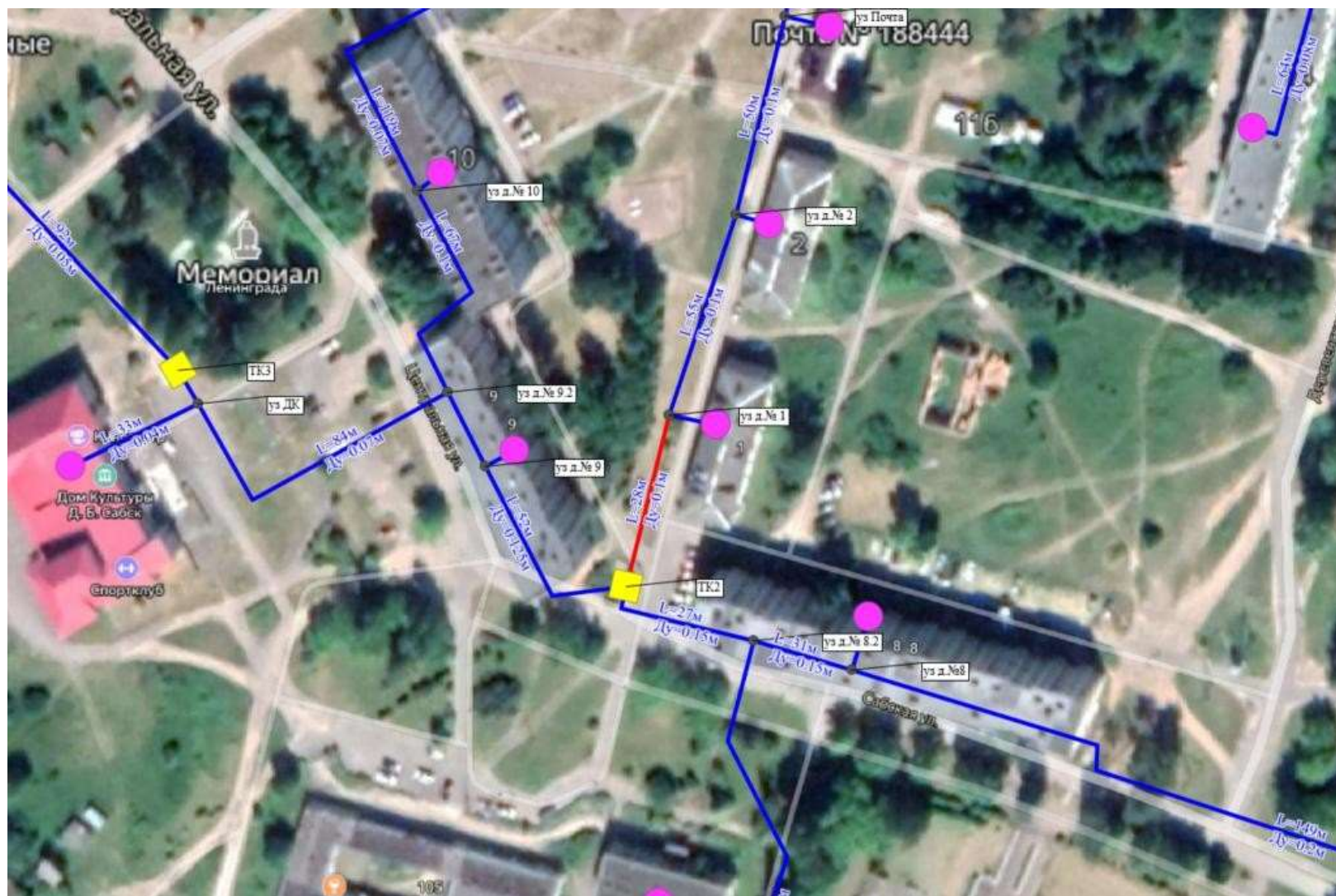
Рисунок 1.3.1 - Отказ подающего трубопровода ДУ 100мм Тк2 – Уз д.№1
